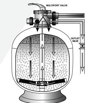
Filtros de fibra de vidrio de montaje superior Waterco
