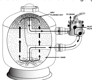
Waterco GFK-Filterkessel mit Seitenanschluss
