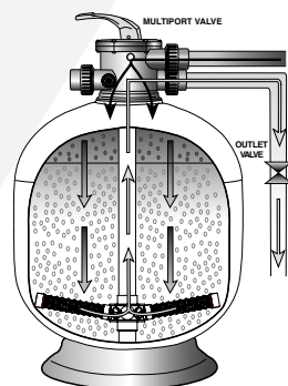
Waterco GFK-Filterkessel mit Obenanschluss
