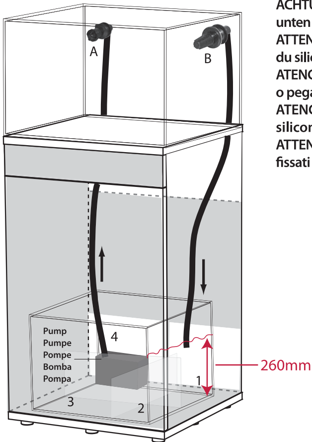
Back view/Rückansicht/Vue arrière Vista posterior/Vista traseira/Vista posteriore
